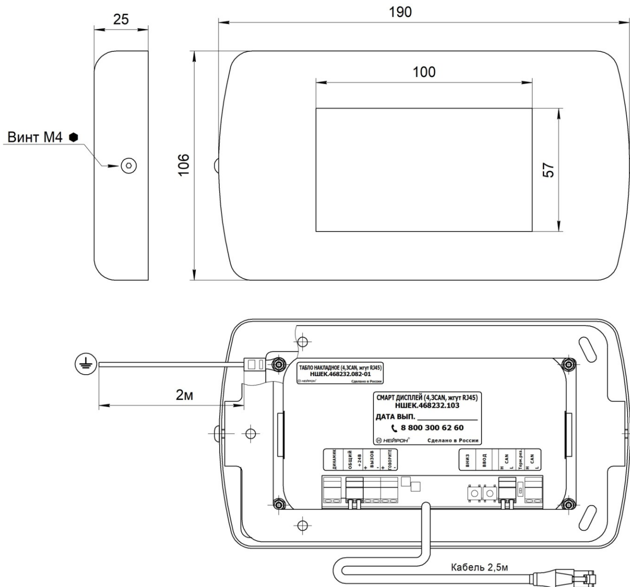
Рис.1 Внешний вид Табло накладное (4,3) НШЕК.468232.082-01
